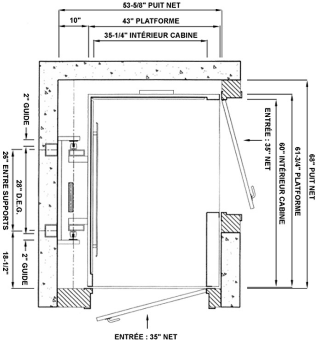
VUE EN PLAN - OP35CE
