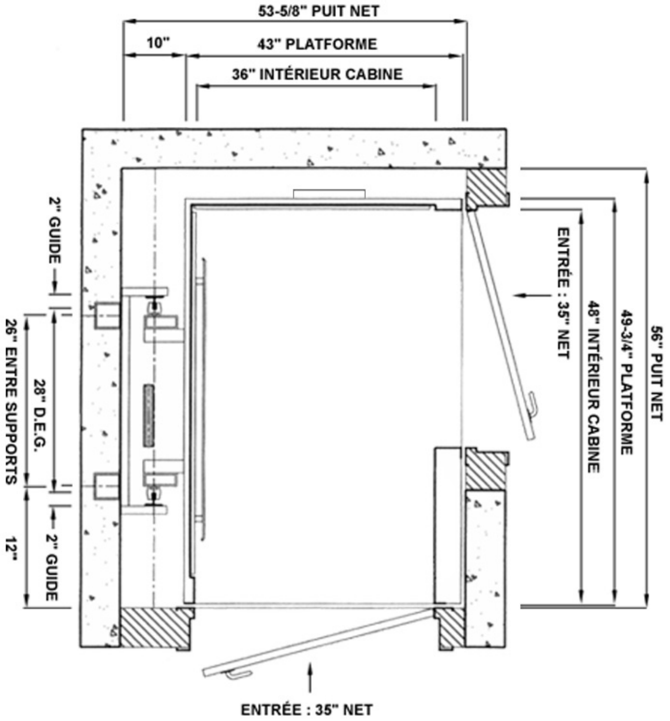
VUE EN PLAN - OP34CE
